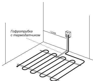
Рис.2 Монтаж датчика температуры пола
