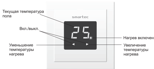
Рис.7 Назначение символов и кнопок
